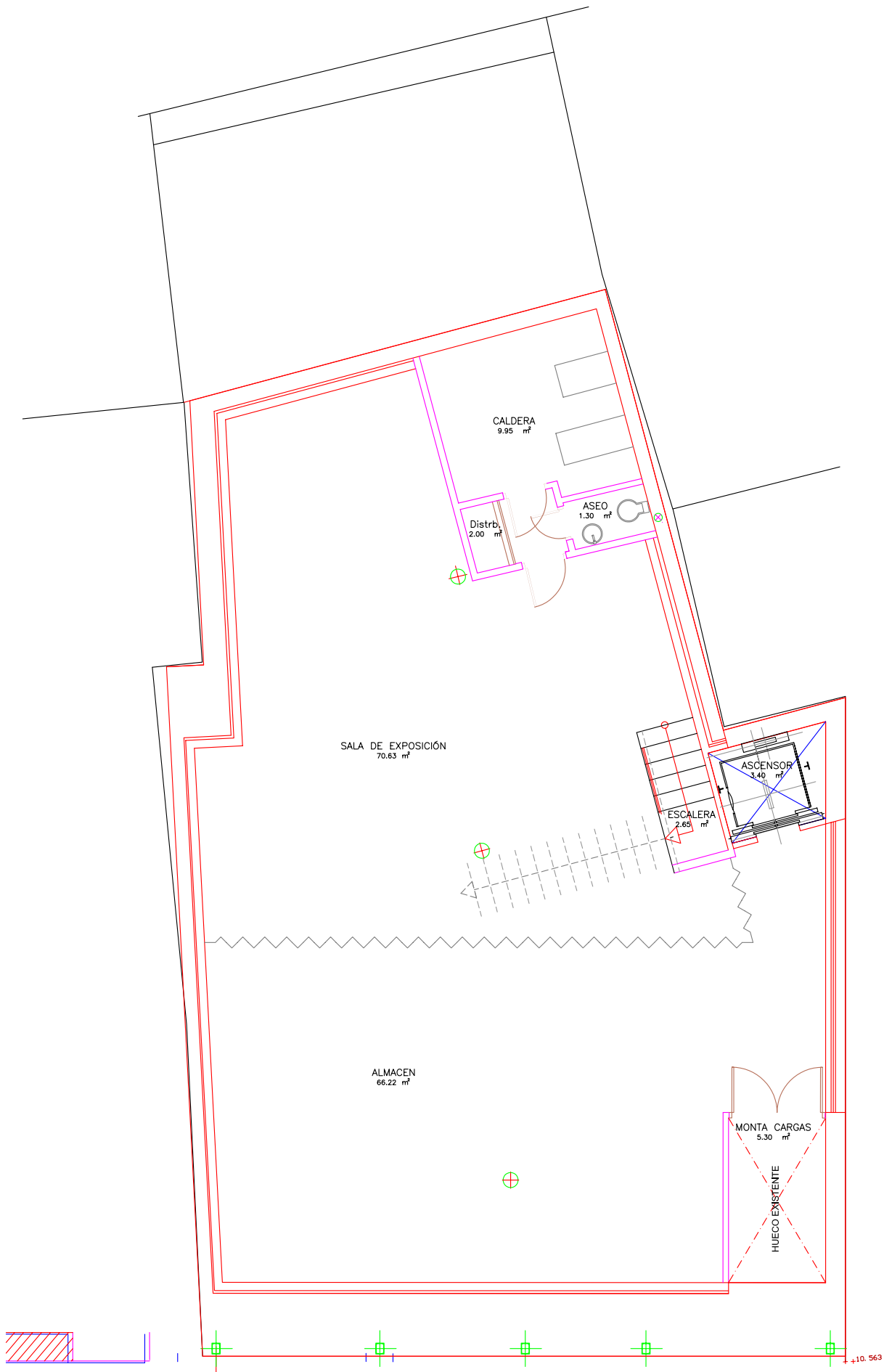
PLANTA SOTANO ESCALA 1/100
